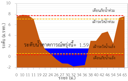
TC221202 สะพานควนโดนโน
