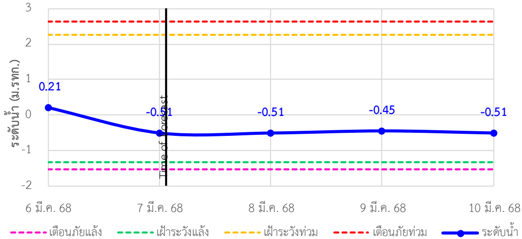
TC221003 สะพานข้ามคลองลำชาน ตำบลย่านตาขาว อำเภอย่านตาขาว จังหวัดตรัง
